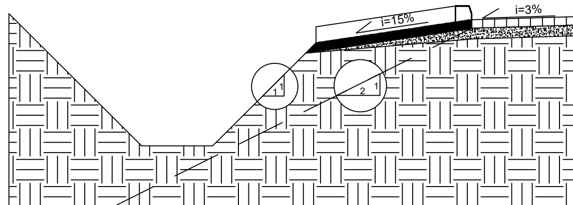
9 Detalhes Entradas para Decida D'água e Sarjeta Sem Escala
