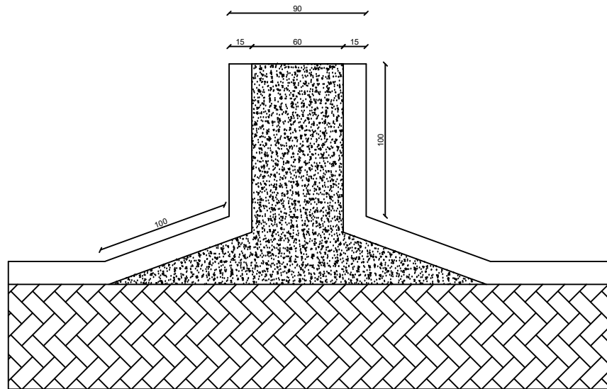
8 Detalhes Entradas para Decida D'água - Vista Superior Sem Escala
